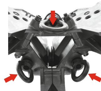
3 Anschlagpunkte
